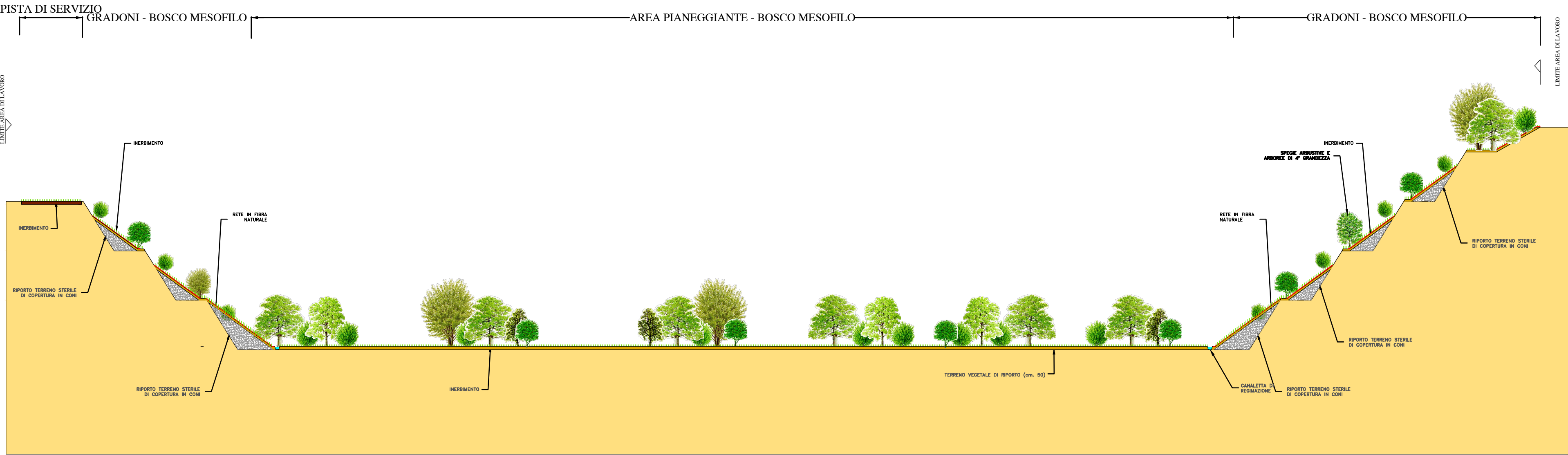
Sezione 2-2
